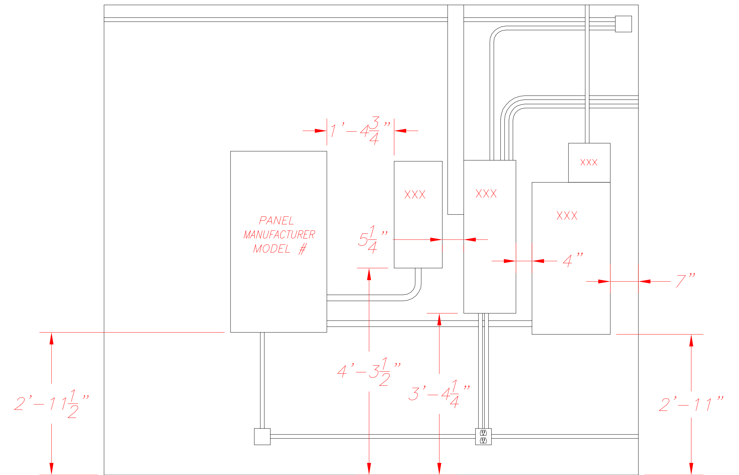
ELEV "B"
